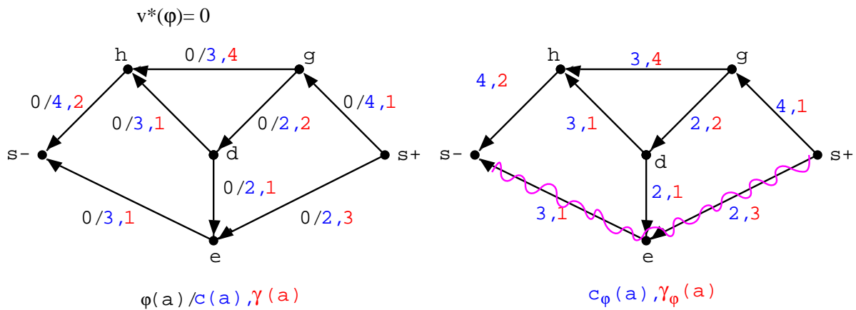
図 2.10: プライマル-デュアル法の動き (最初のフロー \varphi と \mathcal{N}_\varphi の s^+ から s^- への最短路)
