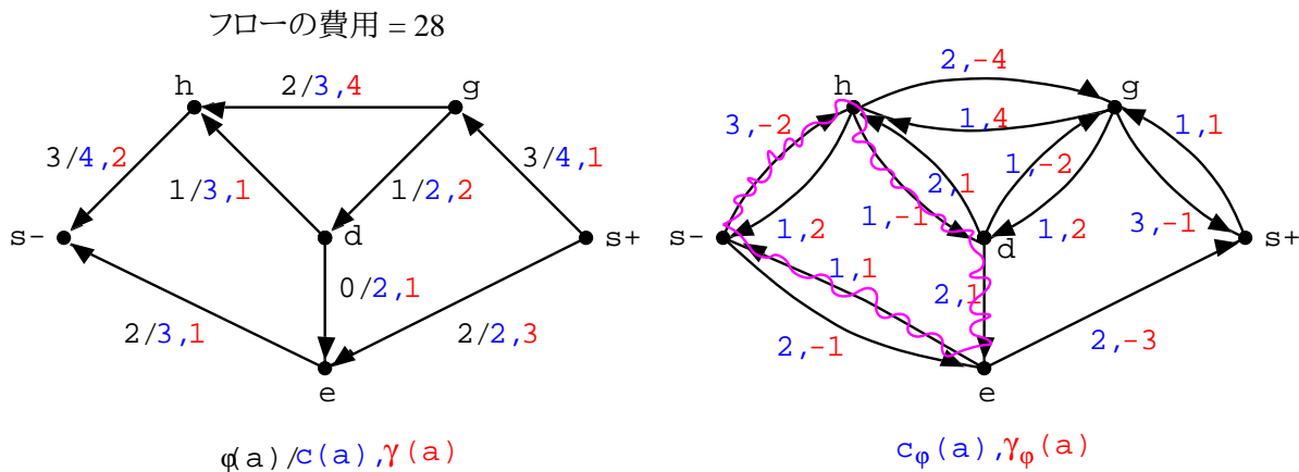
図 2.6: プライマル法の動き (フロー \varphi と, \mathcal{N}_\varphi の有向閉路)
