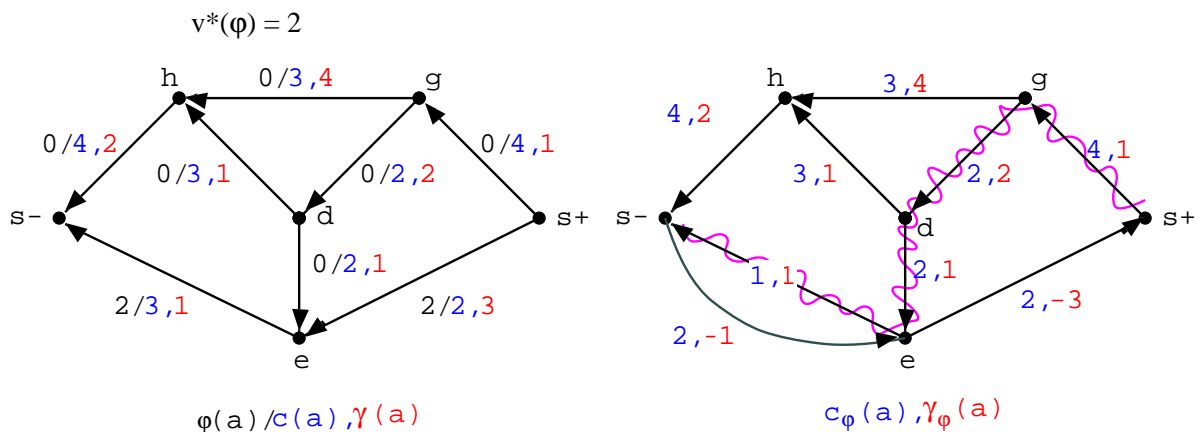
図 2.11: プライマル-デュアル法の動き (フロー \varphi と \mathcal{N}_\varphi の s^+ から s^- への最短路)
