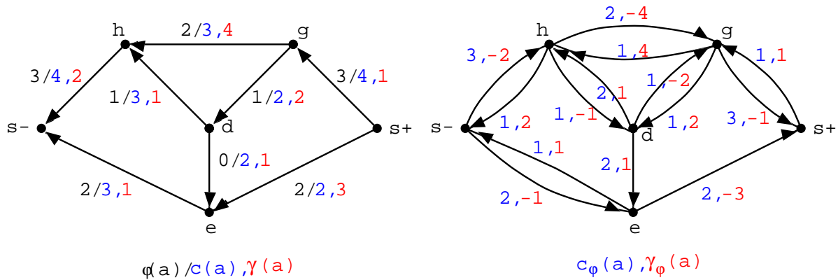
図 2.4: 補助ネットワークの例
