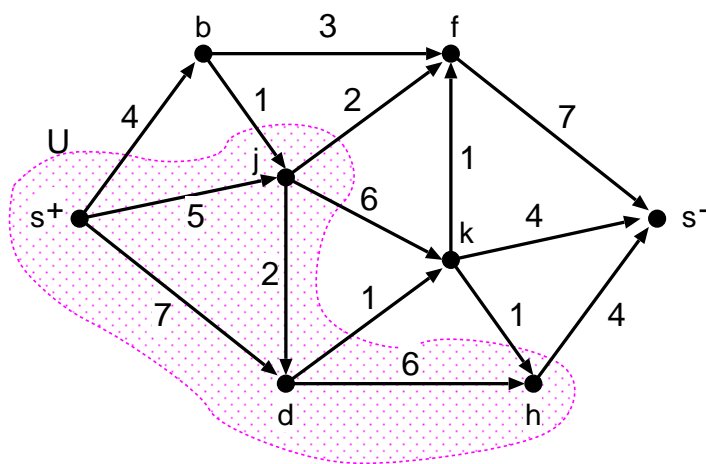
図 2.1: カット U = \{s^+, d, j, h\}
